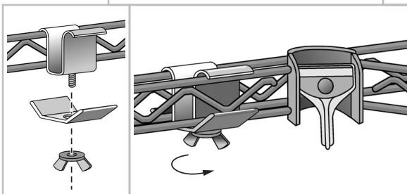
Intermediate S-hook bracket Support de crochet intermédiaire en S Ménsula de gancho doble intermedio
