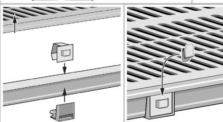
Intermediate S-hook bracket Support de crochet intermédiaire en S Ménsula de gancho doble intermedio
